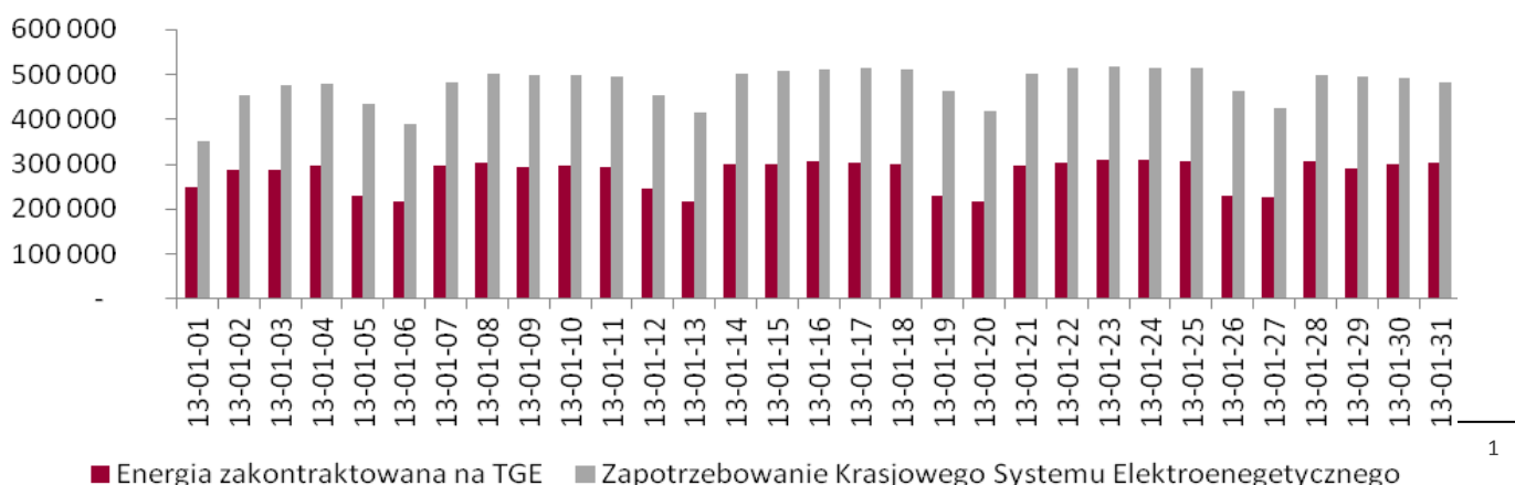
Porównanie wolumenu zakontraktowanej energii elektrycznej na TGE i dziennego łącznego zapotrzebowania KSE w styczniu 2013 roku (MWh)
